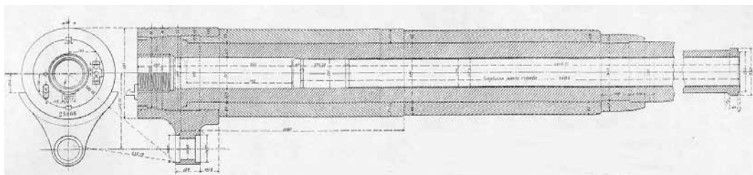
Sezione schematica della bocca da fuoco da 149 A Armstrong per installazione in pozzo
