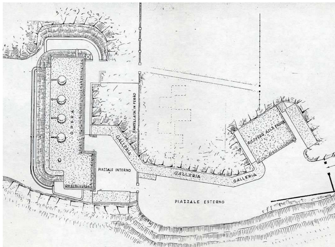
Pianta generale del forte
