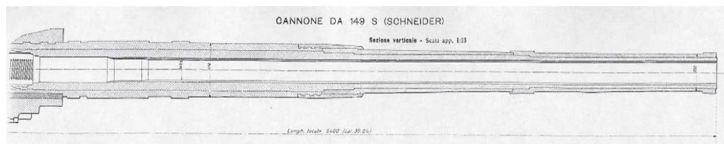
Sezione schematica della bocca da fuoco e dell'otturatore da 149 S
