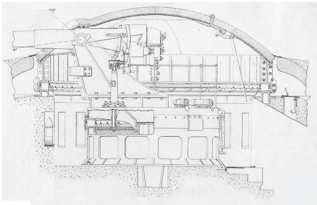
Schema installazione per cannone da 149S in pozzo tipo Schneider
