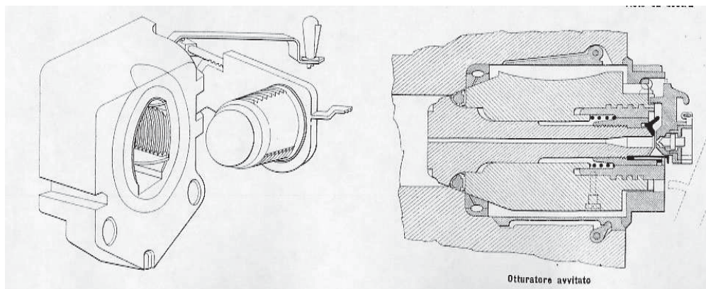
Sezione schematica della bocca da fuoco e dell'otturatore da 149 S
