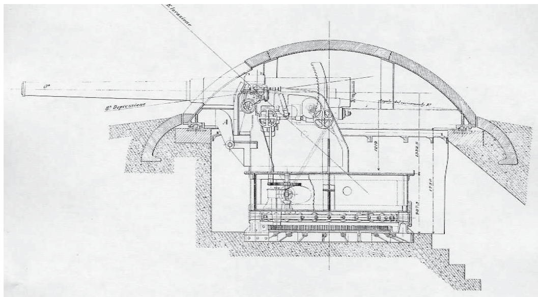
Schema installazione per cannone da 149A in opera a pozzo tipo Armstrong
