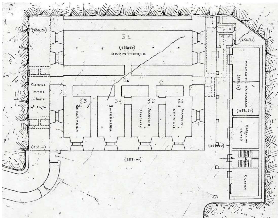
Pianta del ricovero alla prova
